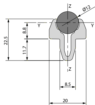
Profilo contenimento tondo Ø12 BPRGD0000020
