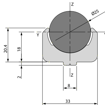
Profilo contenimento tondo Ø25 BPRGD0000022
