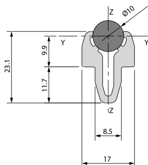
Profilo contenimento tondo Ø10 BPRGD0000032
