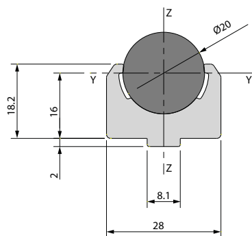
Profilo contenimento tondo Ø20 BPRGD0000021
